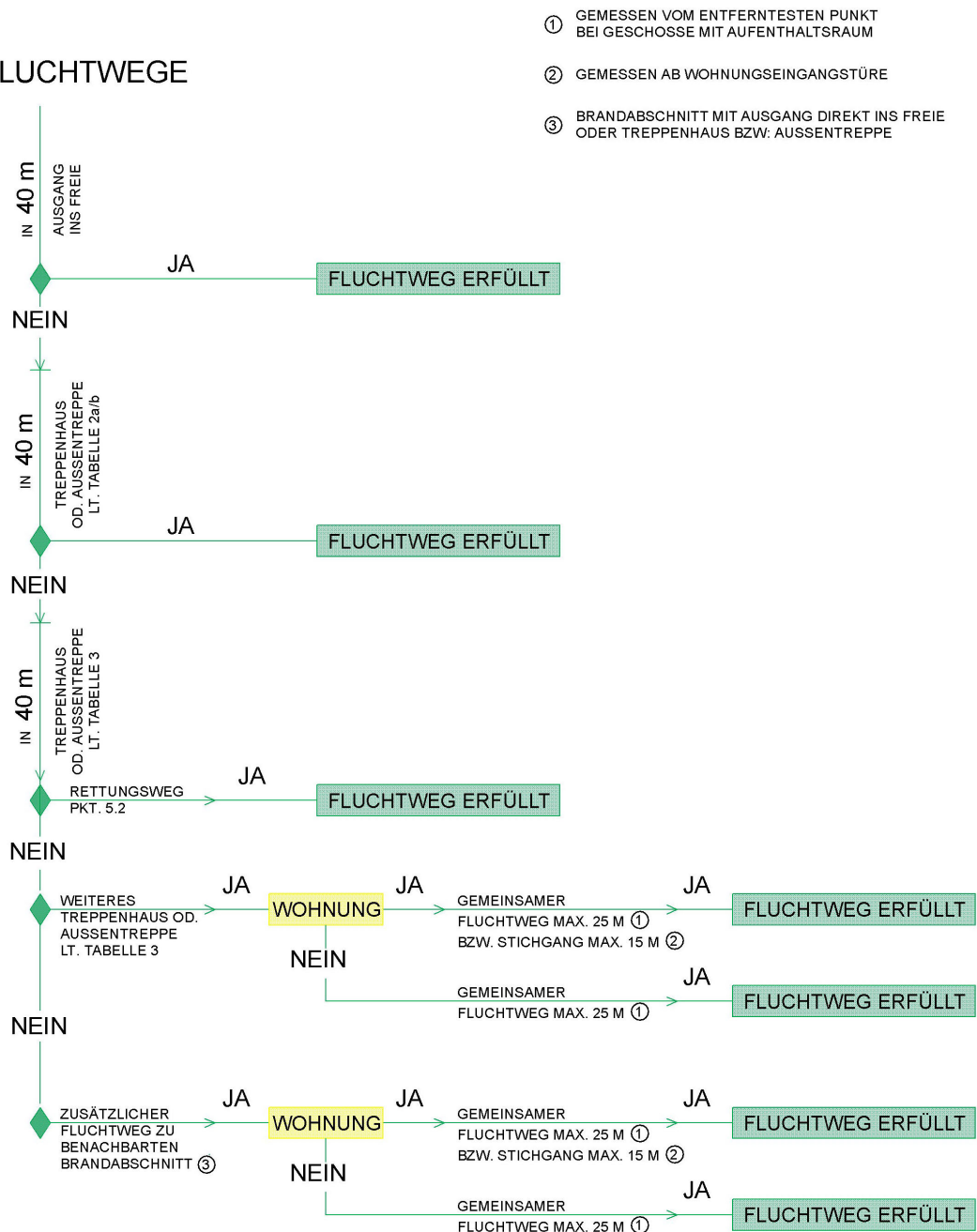
Abbildung 15: zu den Punkten 5.1 und 5.2 – Flucht- und Rettungswege – Ablaufschema
