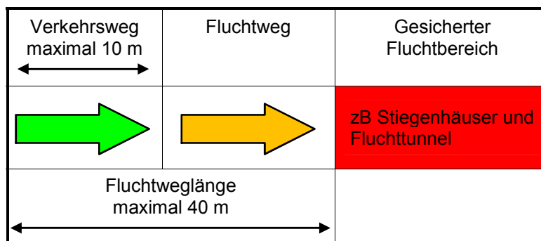
Bild 1 – Fluchtweglänge
