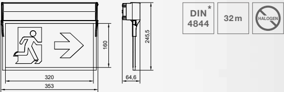
Maßzeichnungen [mm]:
